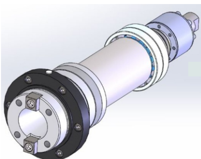
Innenleben SK50
